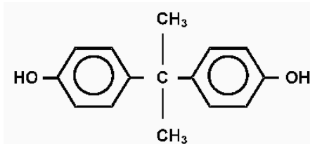
2. ábra Biszfenol A szerkezete
