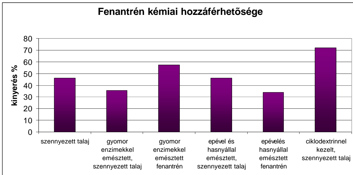
4. ábra: Fenántrén kinyerési hatékonysága különböző előkezelések hatására
