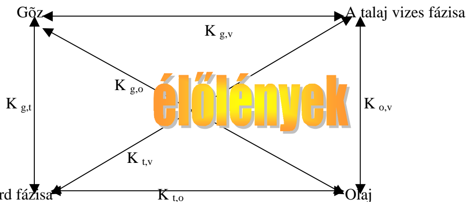
3. ábra: A talaj és a szennyezőanyag fázisainak megoszlása
